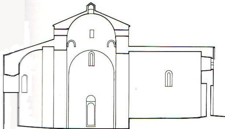
Sant Pere de Graudescales. Secció longitudinal de la nau de l'església (planimetria: J. Segués)
