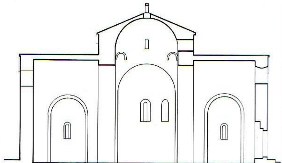
Sant Pere de Graudescales. Secció transversal de la nau de l'església (planimetria: J. Segués)
